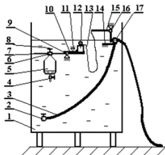
Рисунок 1 – Система автоматичного поливу
