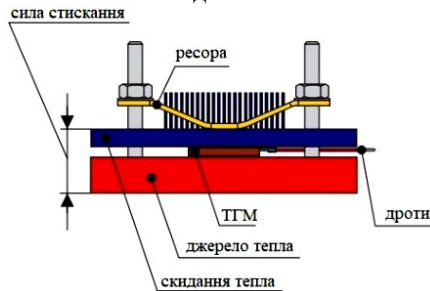
Рисунок 1 – Схема роботи ТЕГ
